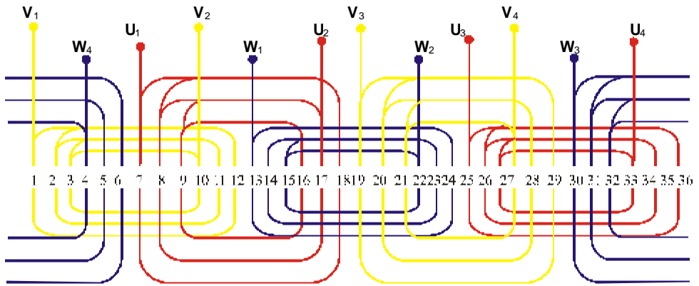
Gambar VI.19 Contoh Belitan Rantai Lapis Tunggal
