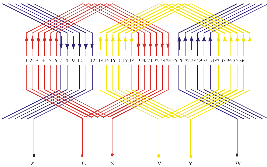
Gambar VI.20 Contoh Belitan Motor Induksi 3 Fasa 36 Alur
