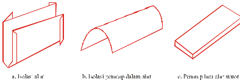
Gambar VI.25 Isolasi Alur Stator
