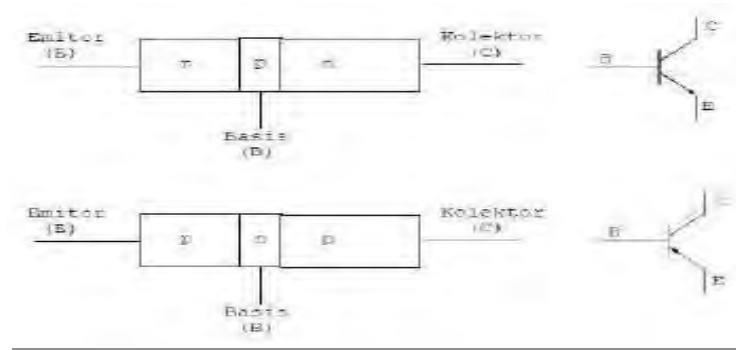
Gambar 4.2 (Konstruksi transistor)
