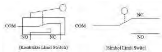
Gambar 3.3 (konstruksi saklar)
