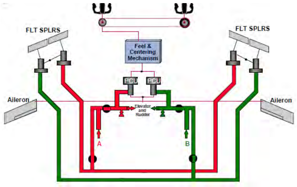
Gambar 9.18(Skema System Hidraulic Pada Aileron)
