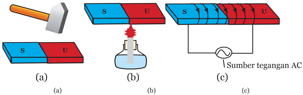
Sumber: Dokumen Kemdikbud Gambar 6.19 Menghilangkan Sifat Magnet dengan Cara (a) Memukul; (b) Memanaskan; dan (c) Meliliti Magnet dengan Arus AC
