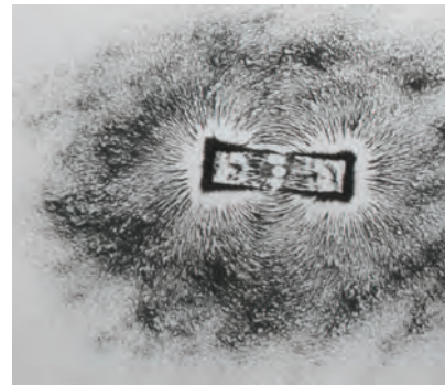
Gambar 6.21 Pola Medan Magnet Batang
