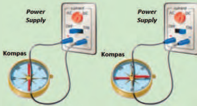
Gambar 6.23 Percobaan Medan Magnet di Sekitar Kawat Berarus
