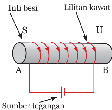
Sumber: Dokumen Kemdikbud Gambar 6.15 Induksi Elektromagnet
