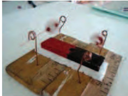
Sumber: Dokumen Kemdikbud Gambar 6.30 Motor Listrik Sederhana
