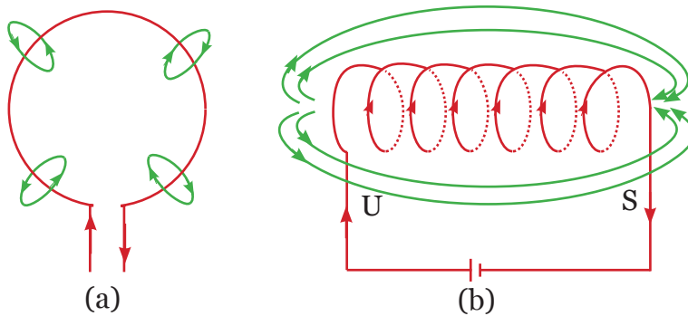
Gambar 6.25 Arah Medan Magnet di Sekitar Kawat Berarus
